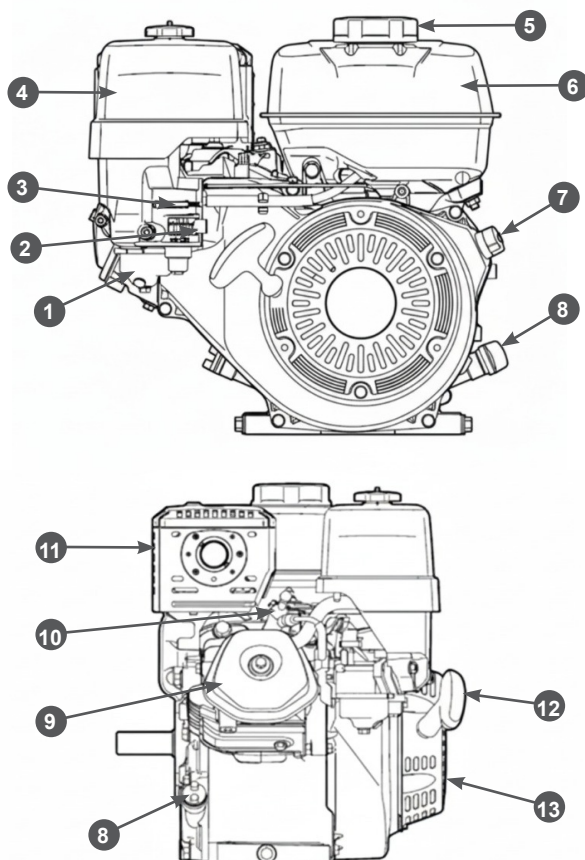
Рис. 2. Основные узлы и органы управления двигателя
