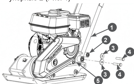
Рис. 4. Установка нижней части рабочей рукоятки
