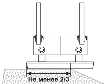
Рис. 15. Расположение виброплиты на краю обрабатываемой поверхности
