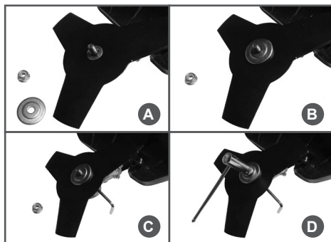
Рис. 9. Установка ножа
