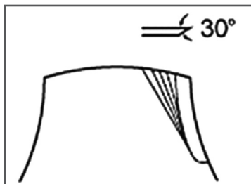
Рис. 20 Заточка ножа
