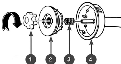
Рис. 13. Снятие триммерной головки
