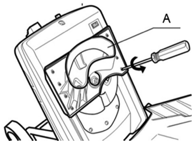
Рис. 8. Снятие защитной пластины
