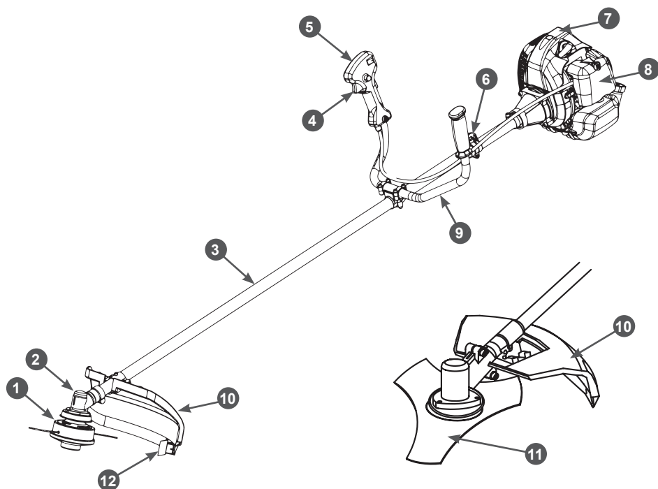
Рис. 1 Основные узлы и органы управления триммера
