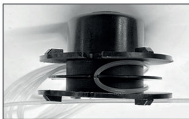
Рис. 23 Установка корда
