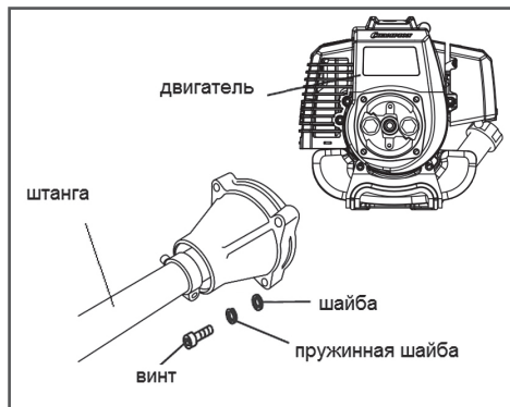
Рис. 6 Соединение двигателя и штанги
