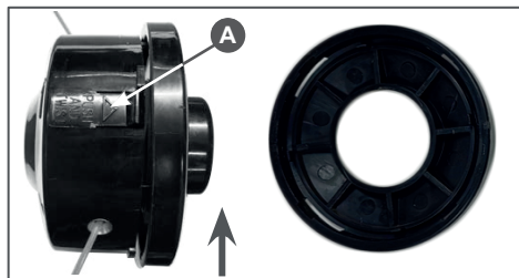
Рис. 22 Снятие крышки триммерной головки
