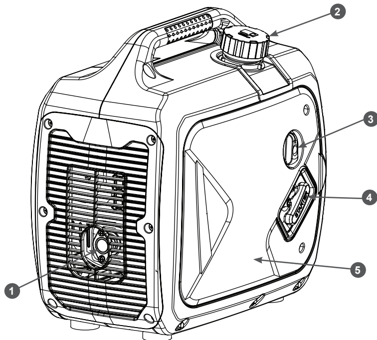
Рис. 2. Основные узлы и органы управления (вид сзади)
