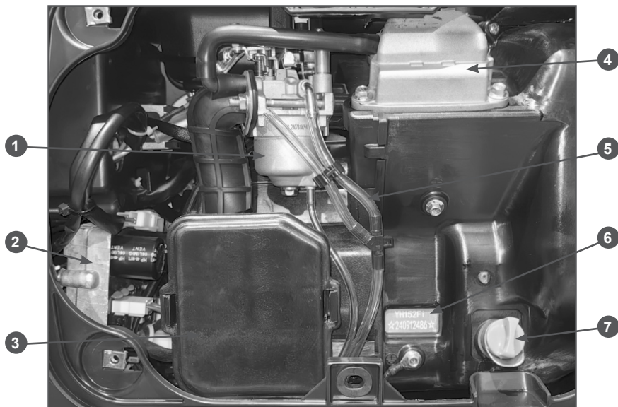
Рис. 3. Основные узлы и органы управления (вид со снятой правой панелью)
