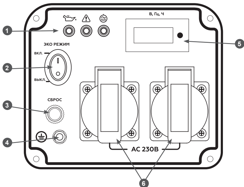
Рис. 4. Панель управления
