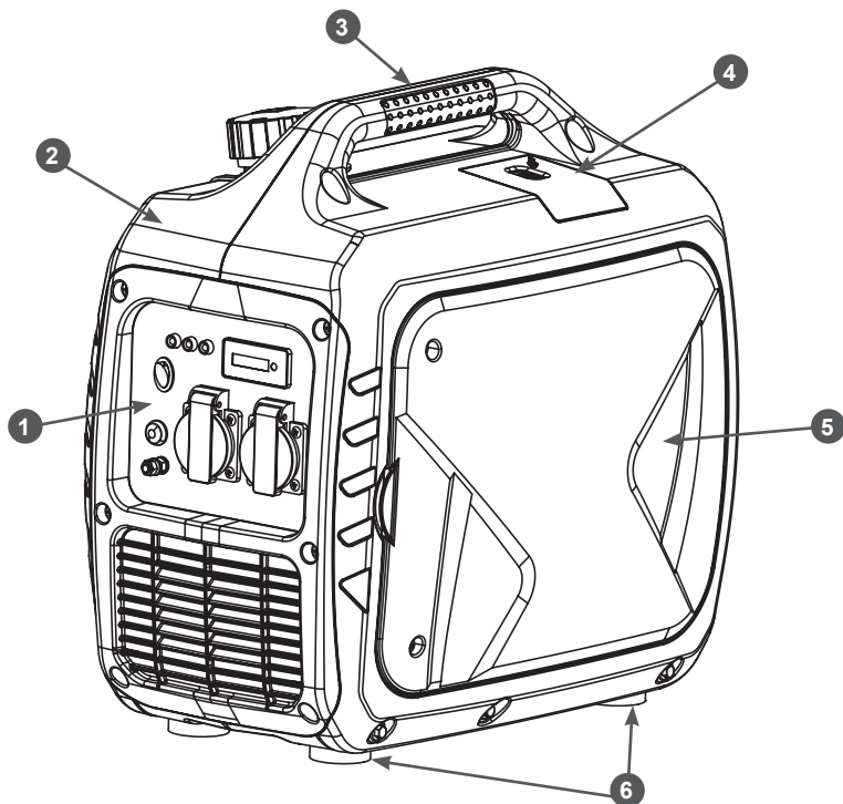
Рис. 1. Основные узлы и органы управления (вид спереди)
