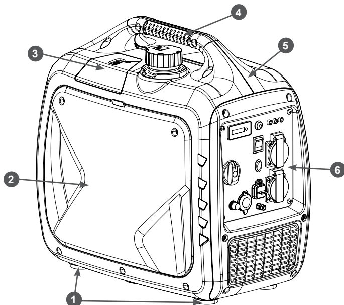
Рис. 1. Основные узлы и органы управления (вид спереди)
