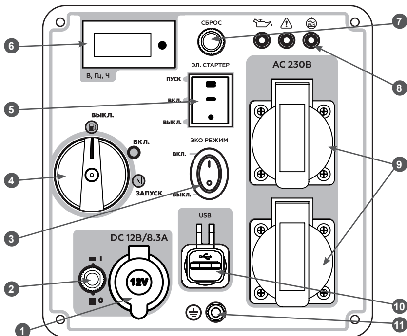
Рис. 4. Панель управления
