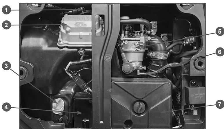
Рис. 3. Основные узлы и органы управления (вид со снятой левой панелью)
