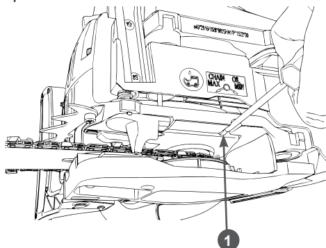
Рис. 13 Регулировка подачи масла на цепь.
