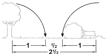
Рис. 18. Рабочая зона вокруг оси дерева
