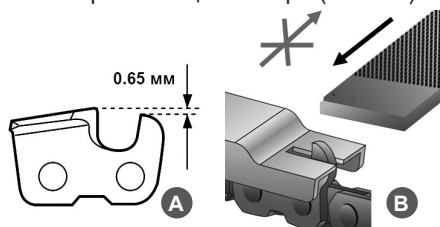
Рис. 36. Проверка высоты ограничителя глубины резания
