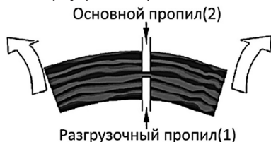
Рис. 23. Распиливание дерева, когда его верхняя часть находится под напряжением
