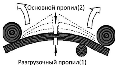
Рис. 26. Распиливание дерева, когда оба конца дерева зажаты и находятся под напряжением
