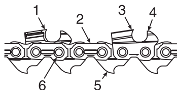
Рис. 33. Конструкция пильной цепи
