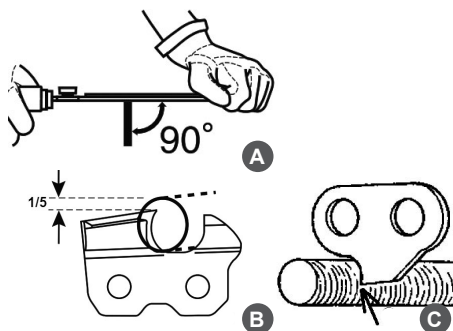
Рис. 35. Положение напильника при заточке
