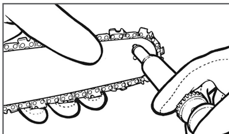
Рис. 38. Смазывание подшипника ведомой звездочки шины
