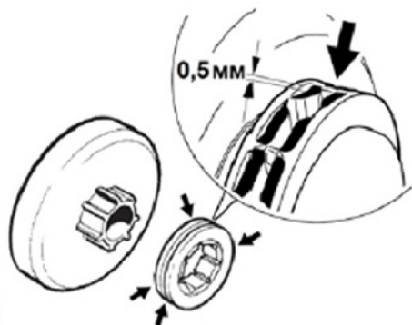
Рис. 40. Максимально допустимая глубина износа зубцов сменного венца
