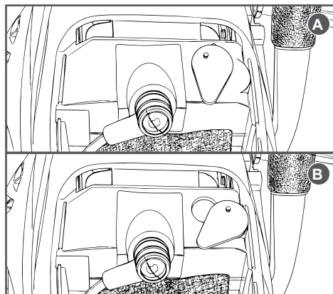
Рис. 15. Положение заслонки обогрева карбюратора
