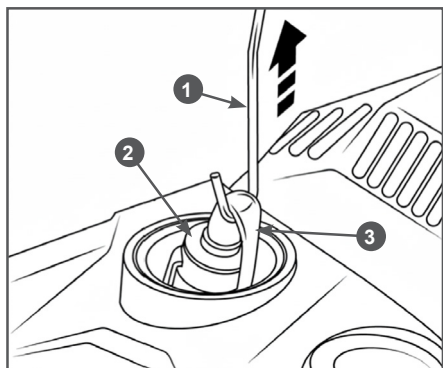
Рис. 28. Обслуживание топливного фильтра
