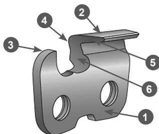
Рис. 37. Части режущего звена цепи
