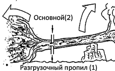
Рис. 25. Распиливание дерева, когда толстый ствол с комлевой частью находится под напряжением
