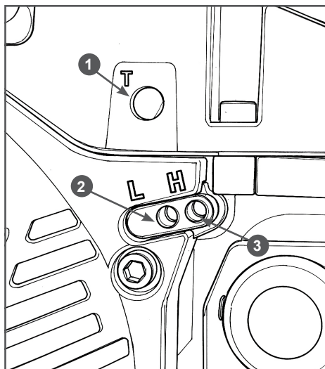
Рис. 31. Винты регулировки карбюратора.
