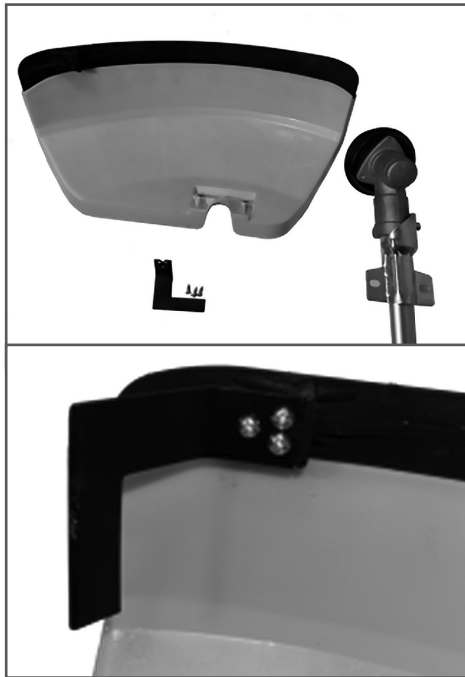
Рис. 2 Установка ножа для обрезки корда
