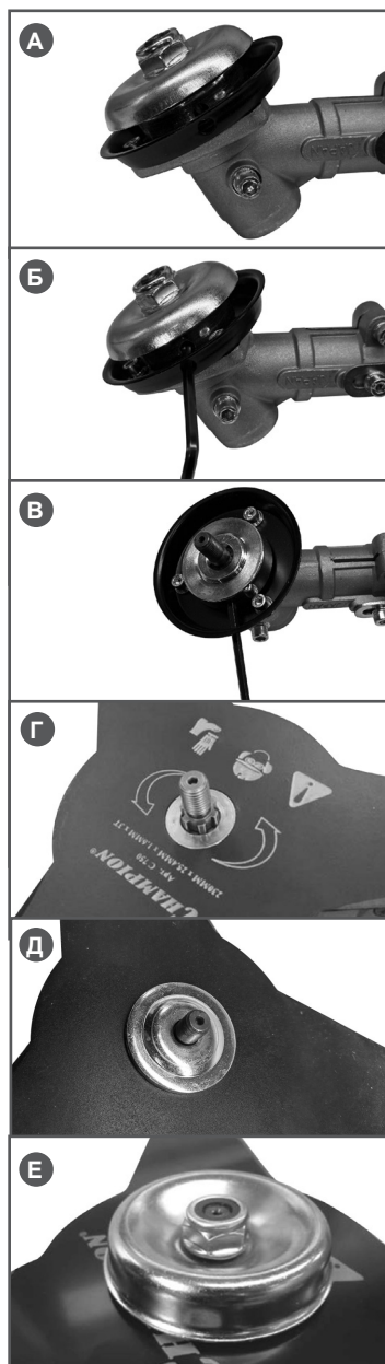
Рис. 4 Установка ножа
