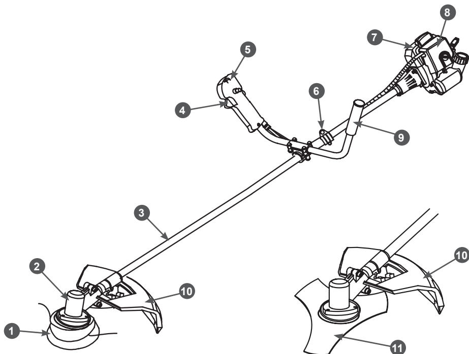
Рис. 1 Основные узлы и органы управления триммера
