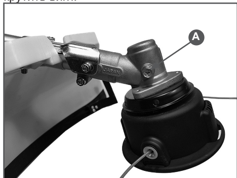
Рис. 20 Винт отверстия для заправки
