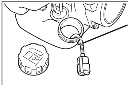
Рис. 18 Обслуживание топливного фильтра
