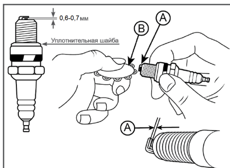
Рис. 19 Проверка зазора между электродами
