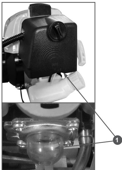
Рис. 9 Расположение ручного топливного насоса
