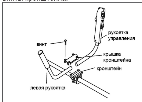
Рис. 7 Установка рукояток
