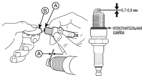
Рис. 38. Проверка межэлектродного зазора А – зазор В – щуп
