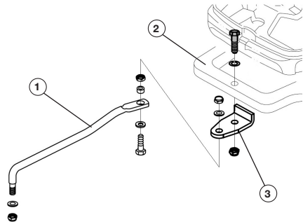
Рис. 15 Установка рулевой тяги
