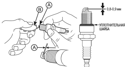
Рис. 49 Проверка зазора между электродами
