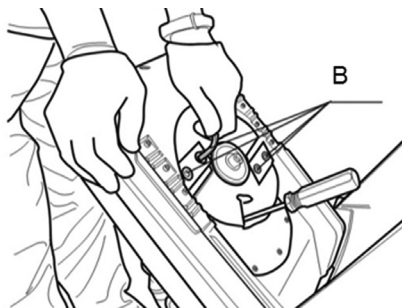
Рис. 8. Снятие ножей
