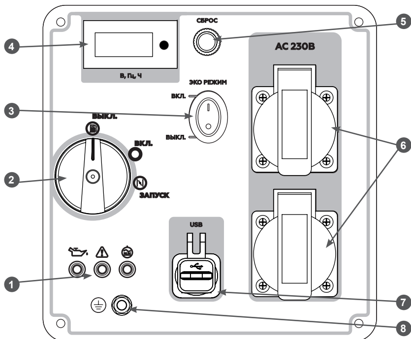
Рис. 4. Панель управления
