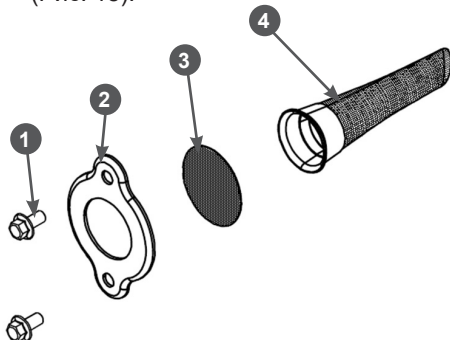
Рис. 18. Обслуживание искрогасителя
