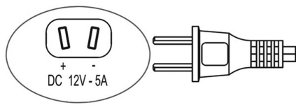
Рис. 9 Розетка 12В
