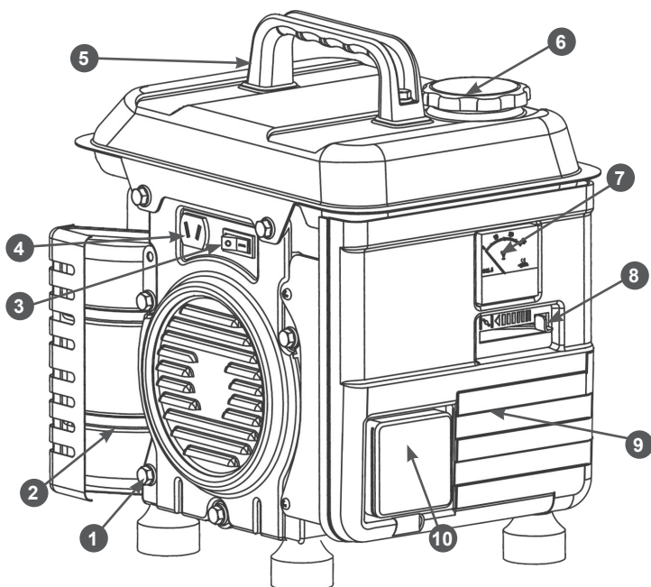
Рис. 1 Расположение основных узлов и органов управления генератора (вид спереди)
