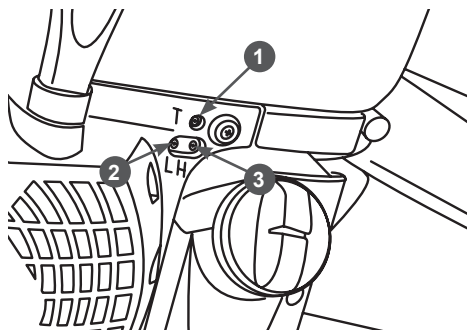
Рис. 19 Виты регулировки карбюратора 1 - винт «Т», 2 - винт «L», 3 - винт «H»
