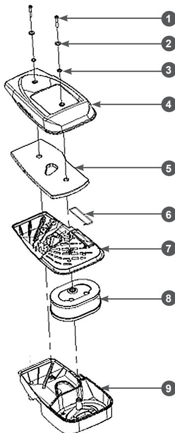
Рис. 17 Воздушный фильтр
