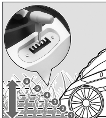
Рис. 8 Регулировка высоты кошения
