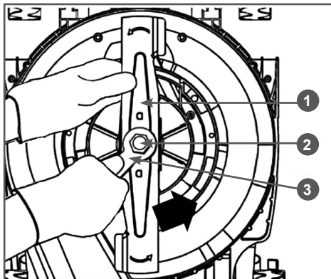
Рис. 13 Замена ножа
