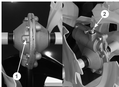
Рис. 44 Добавление смазки в редуктор
