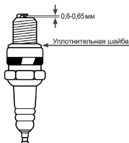
Рис. 11 Свеча зажигания
