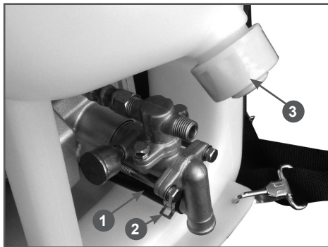
Рис. 8 Крышка сливного отверстия и шланг насоса
