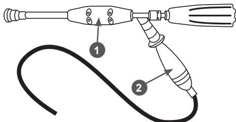
Рис. 2 Присоединение пистолета-распылителя
