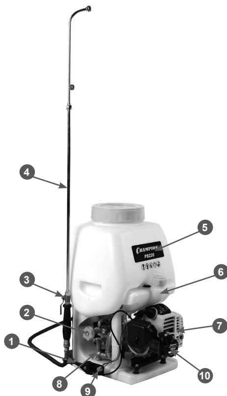
Рис. 1 Основные узлы и органы управления
