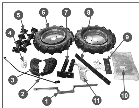
Рис. 2 Комплектация мотоблока
