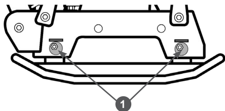
Рис. 22 Замена ремня вибратора 1. Шайбы эксцентриковые (4 шт.)
