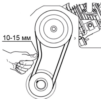
Рис. 21 Проверка натяжения ремня привода вибратора
