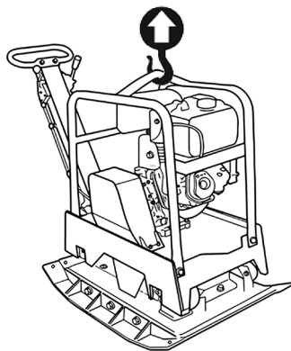
Рис. 23 Точка зацепа крюка подъемного устройства
