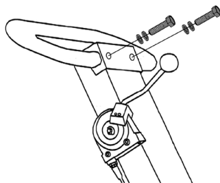
Рис. 3 Установка рабочей рукоятки
