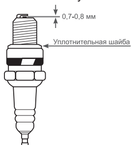
Рис. 19 Обслуживание свечи зажигания
