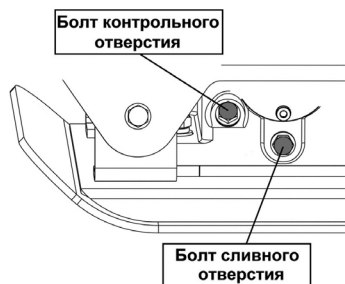
Рис. 20 Отверстия для заправки и слива масла
