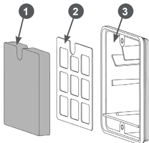
Рис. 13 Обслуживание воздушного фильтра
