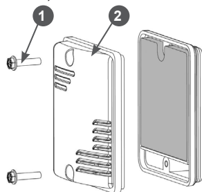
Рис. 12 Снятие крышки воздушного фильтра
