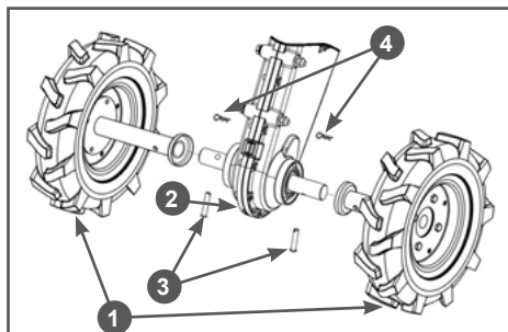
Рис. 8 Установка колес
