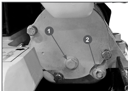
Рис. 22 Замена масла в вибраторе
