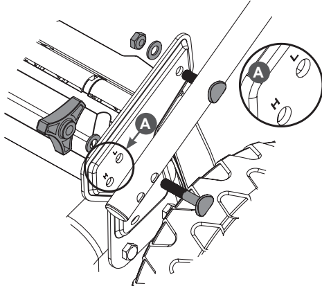
Рис. 4. Установка нижней части рукоятки
