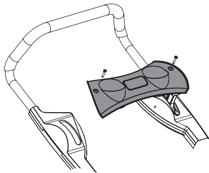
Рис. 10. Установка панели с подстаканниками
