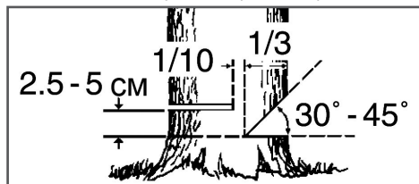
Рис. 14 Расположение запила и пропила
