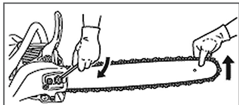
Рис. 4 Затяжка гаек крепления шины
