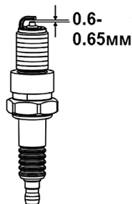
Рис.17 Свеча зажигания
