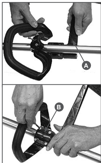
Рис. 4 Установка рабочей рукоятки
