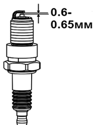
Рис.14 Свеча зажигания
