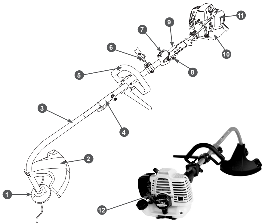
Рис.1 Расположение основных узлов и органов управления
