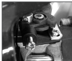
Рис.13 Винт настройки оборотов холостого хода
