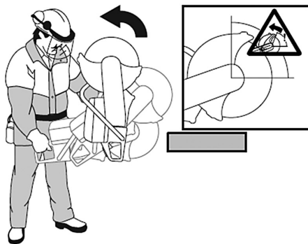
Рис. 12 Движение бензореza при отдаче
