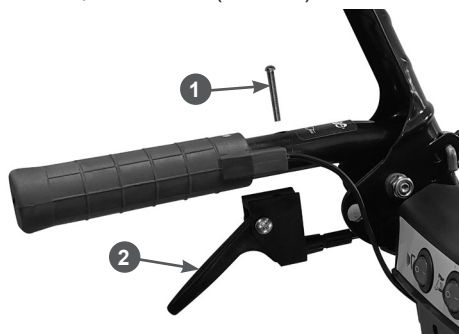
Рис. 14 Установка рычага поворота 1. Болт 2. Рычаг
