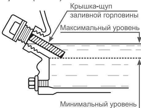
Рис. 29 Проверка уровня масла по щупу нижней маслосазливной горловины
