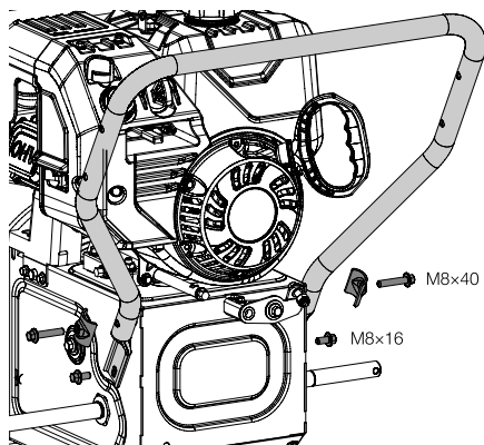
Рис. 5. Установка стойки рукояток
