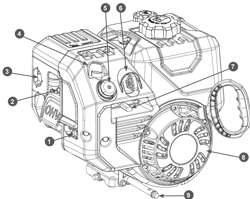
Рис. 3. Основные узлы и органы управления двигателя (вид со стороны стартера)
