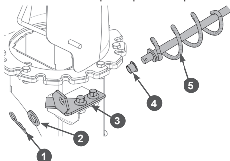
Рис. 14. Установка рычага управления поворотом жёлоба (сторона жёлоба)
