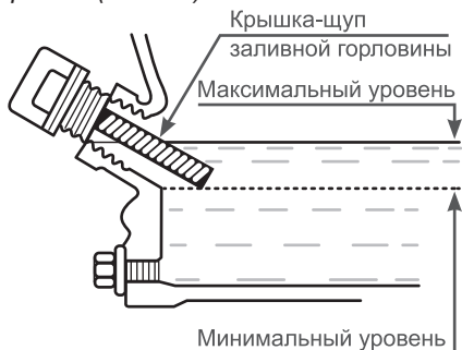
Рис. 17. Проверка уровня масла по щупу нижней маслозаливной горловины
