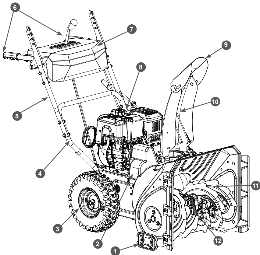
Рис. 1. Основные узлы и органы управления (вид спереди)
