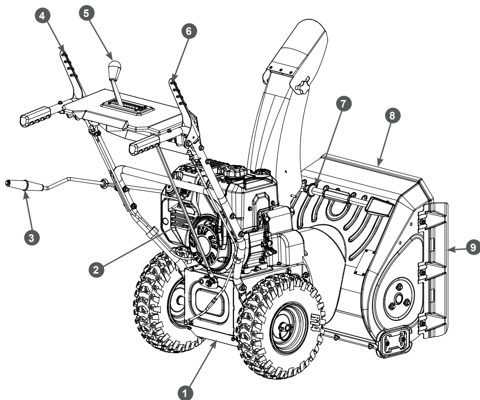
Рис. 2. Основные узлы и органы управления (вид сзади)
