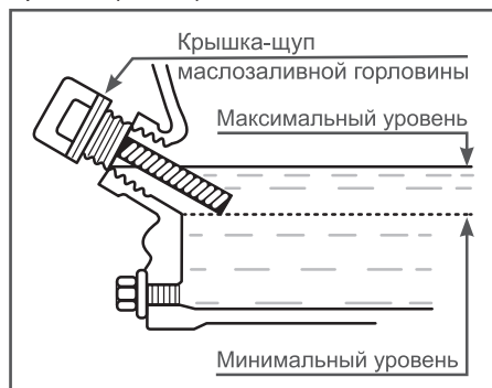
Рис. 8 Проверка уровня масла в картере 6. Плотнo закрутите крышку-щуп.
