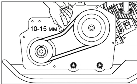
Рис. 27 Проверка натяжения ремня
