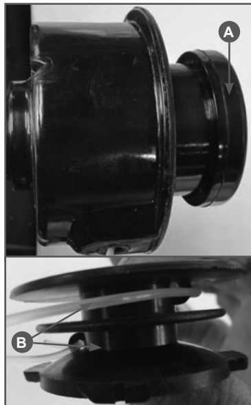
Рис. 10 Снятие крышки триммерной головки
