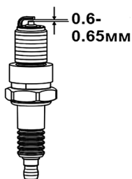
Рис.14 Свеча зажигания
