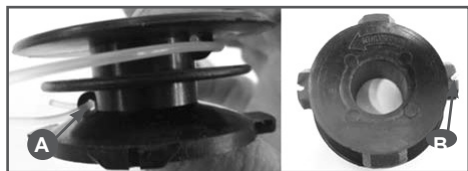
Рис. 24 Установка корда
