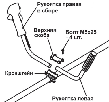
Рис. 6 Установка рукояток
