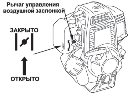
Рис. 11 Рычаг управления воздушной заслонкой
