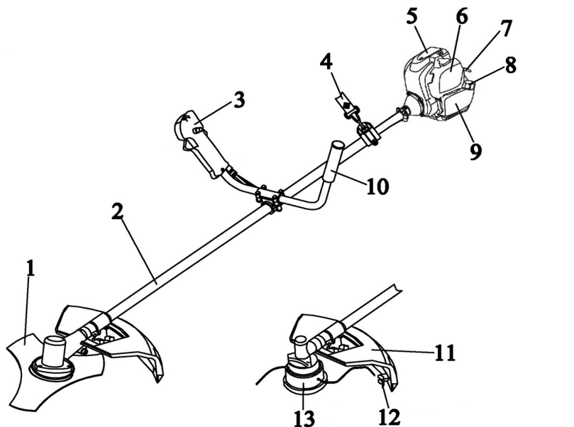
Рис. 1 Основные узлы и органы управления
