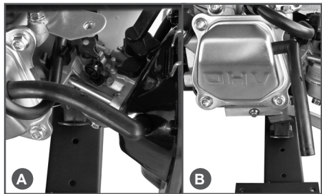
Рис. 12 Трубка сапуна
