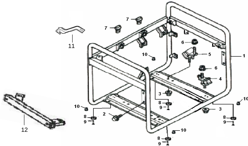
( Frame )
