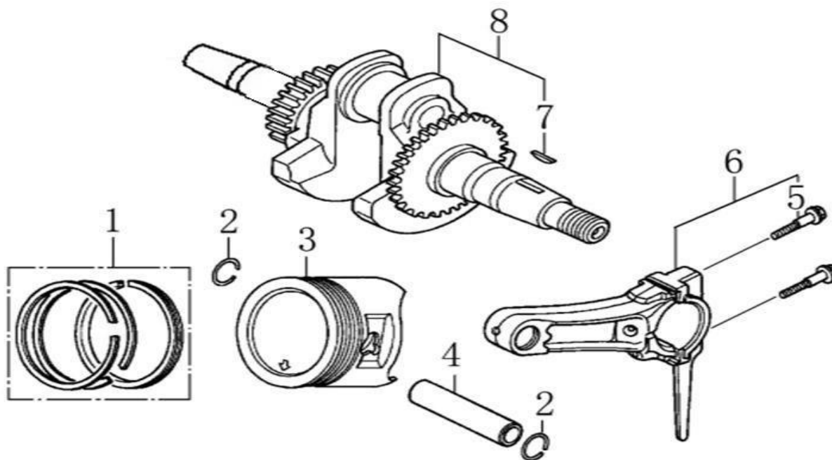
( CRANKSHAFT/PISTON)
