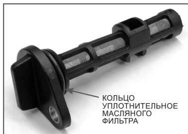
Рис. 19 Масляный фильтр
